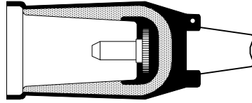
BIF-B-24 ENS.3 Bouchon Isolant Femelle Code : 96780 - Codet EDF: 67.94.205
