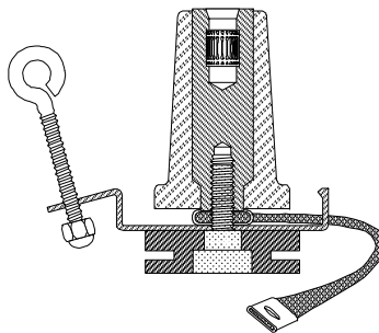
PMT-B-24 ENS.3 Plot de Mise à la terre Code : 96779 Codet EDF 67.94.202
